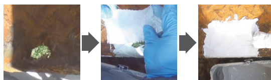
鉄骨階段に空いた穴 ガラスクロスを貼り付けて 上から塗布して補修・補強が完了!
